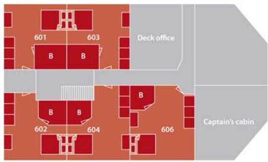
E-deck 6
